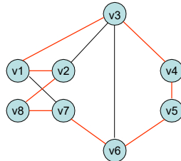
Hamiltonian Circuit {v1,v2,v8,v7,v6,v5,v4,v3,v1}
